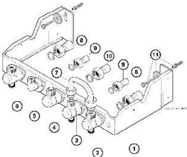
Fig. 7 Placa de racorduri
